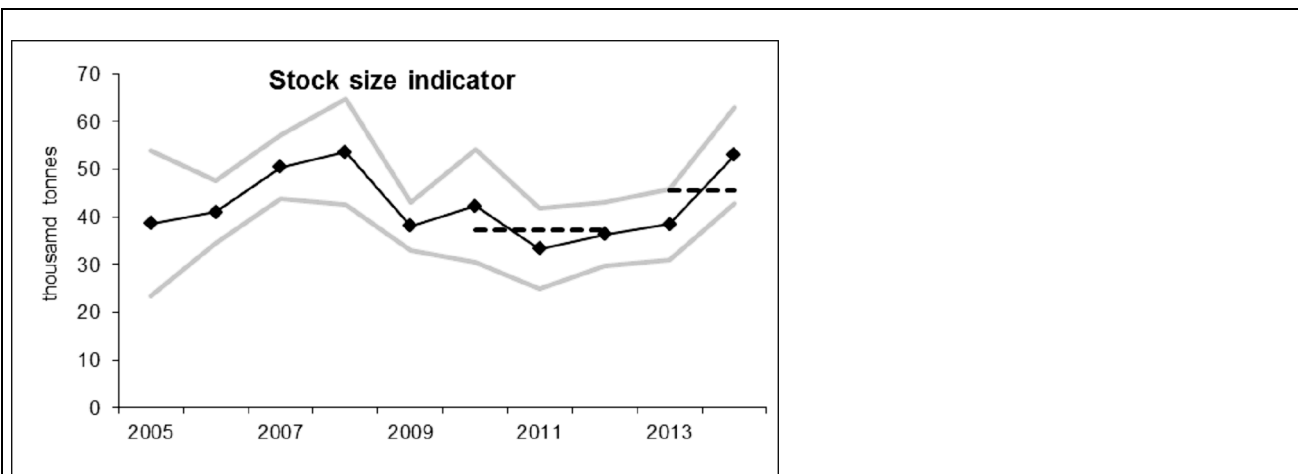
Evolution de l'indice de biomasse moyen (campagnes irlandaise et écossaise en IV et VI)
